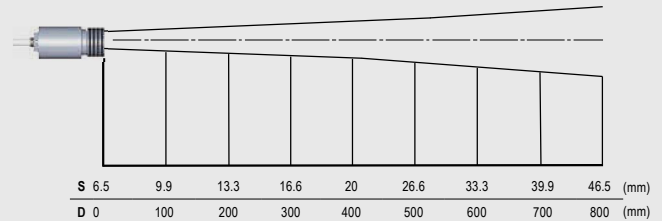
20:1 optics
