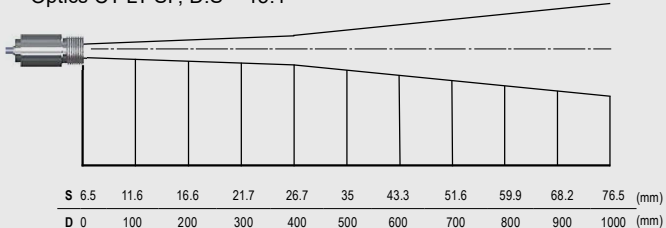
Optics CT LT SF, D:S = 15:1
