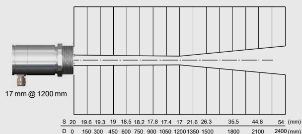
Chart SF optics, D:S = 70:1
